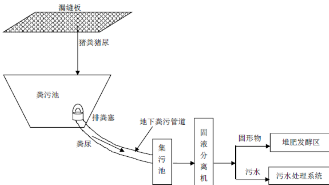
图3-2 项目猪场干清粪工艺示意图
