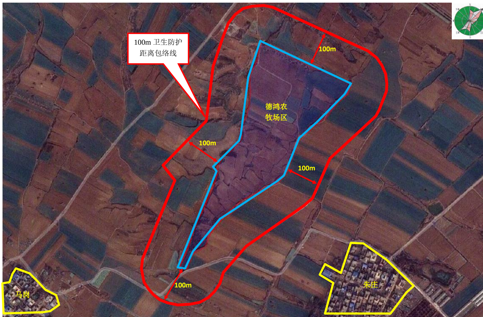
附图八 项目场区卫生防护距离包络线图
