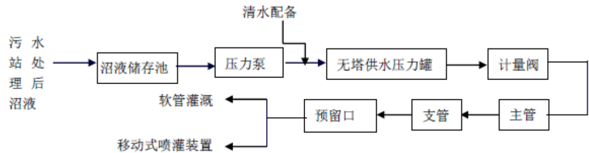
图6-6 沼液农田利用流程图
