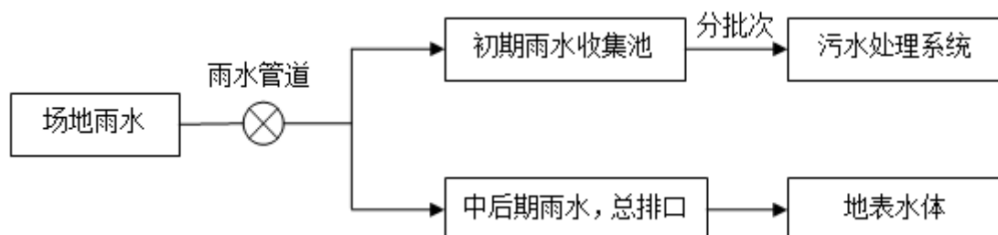
图3-6 本工程初期雨水收集和排放示意图
