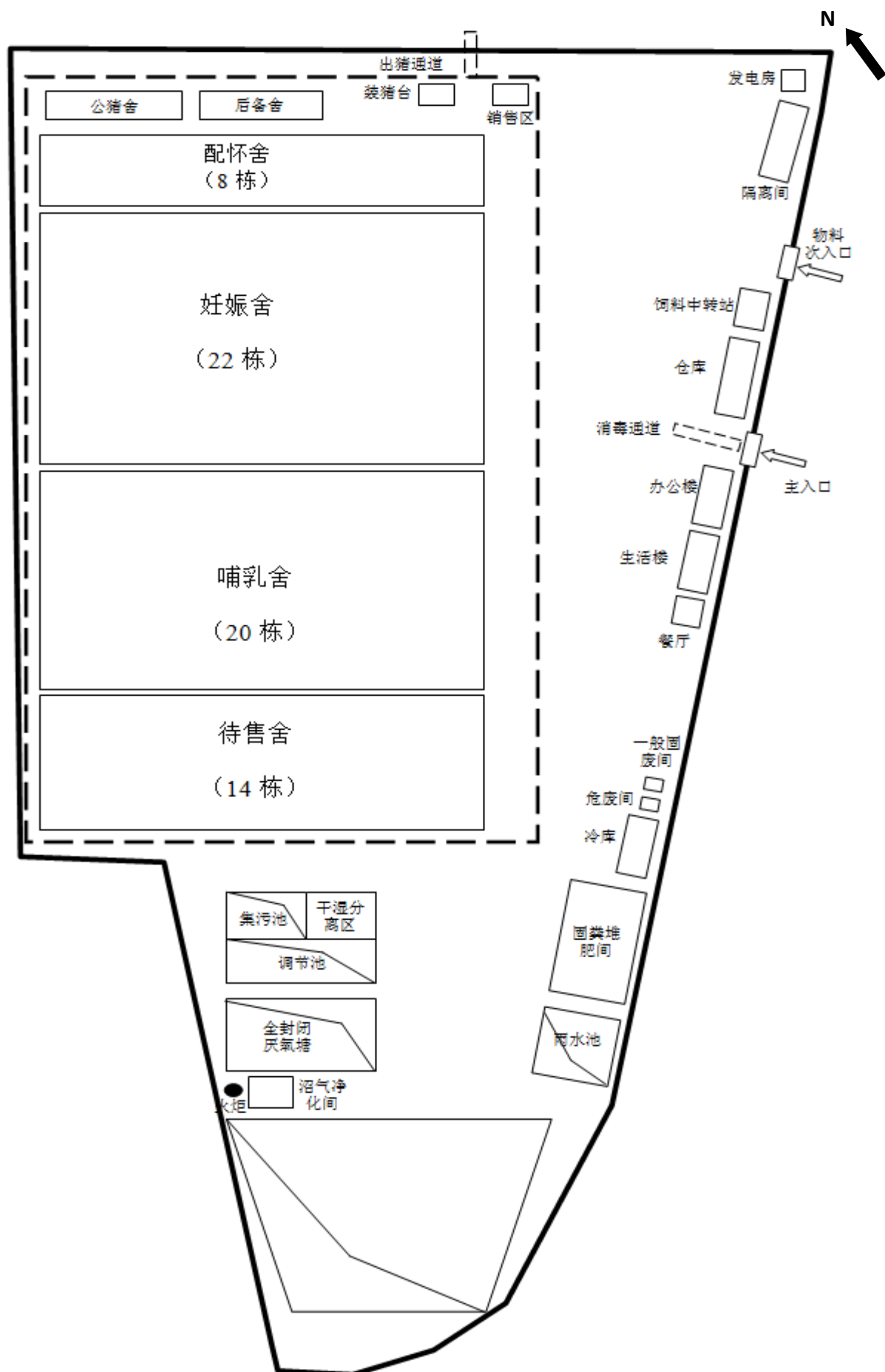
附图四 项目场区平面布置图
