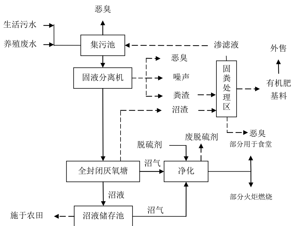
图6-2 本项目废水处理工艺流程及产污环节图
