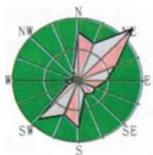
图4-1 唐河县全年风频玫瑰图
