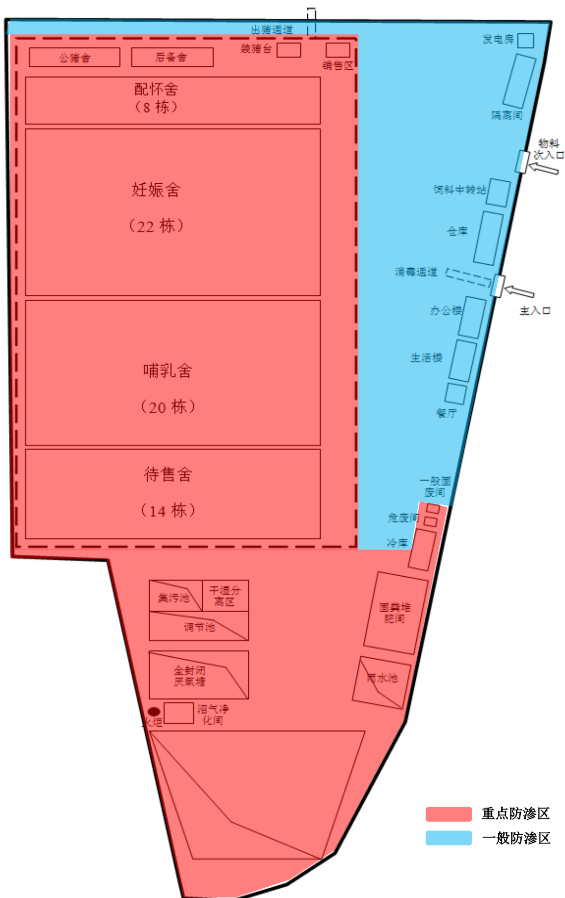
附图七 项目场区地下水分区防渗分布图
