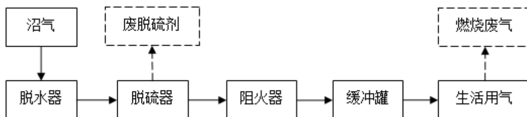
图3-4 沼气利用流程及产污环节示意图
