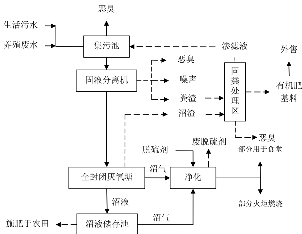
图3-3 项目粪污处理工艺流程及产污环节示意图
