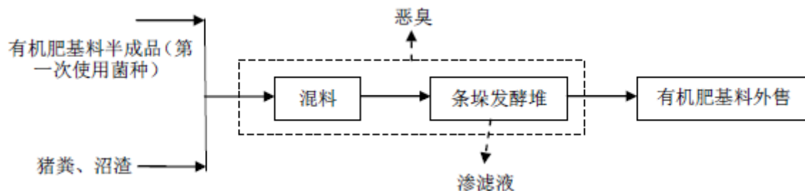
图 3-5 本项目有机肥基料工艺流程及产污环节图
