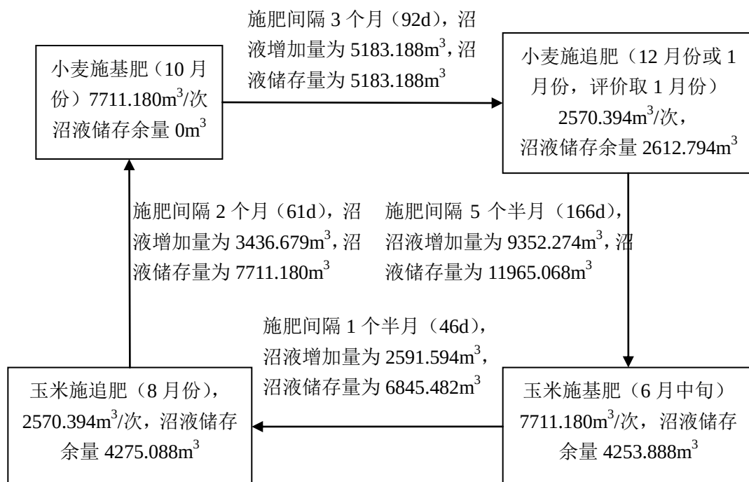
图6-7 沼液全年田间施肥平衡图
