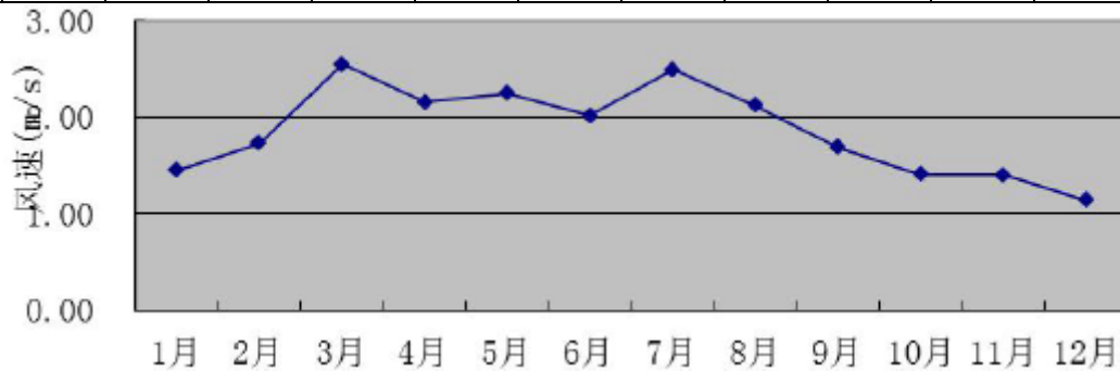
图5-2 唐河县2019年年平均风速月变化图
