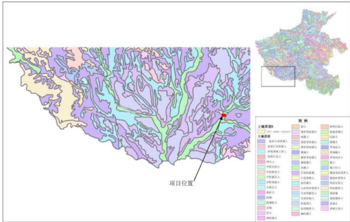
图 5-11 项目区域土壤类型
