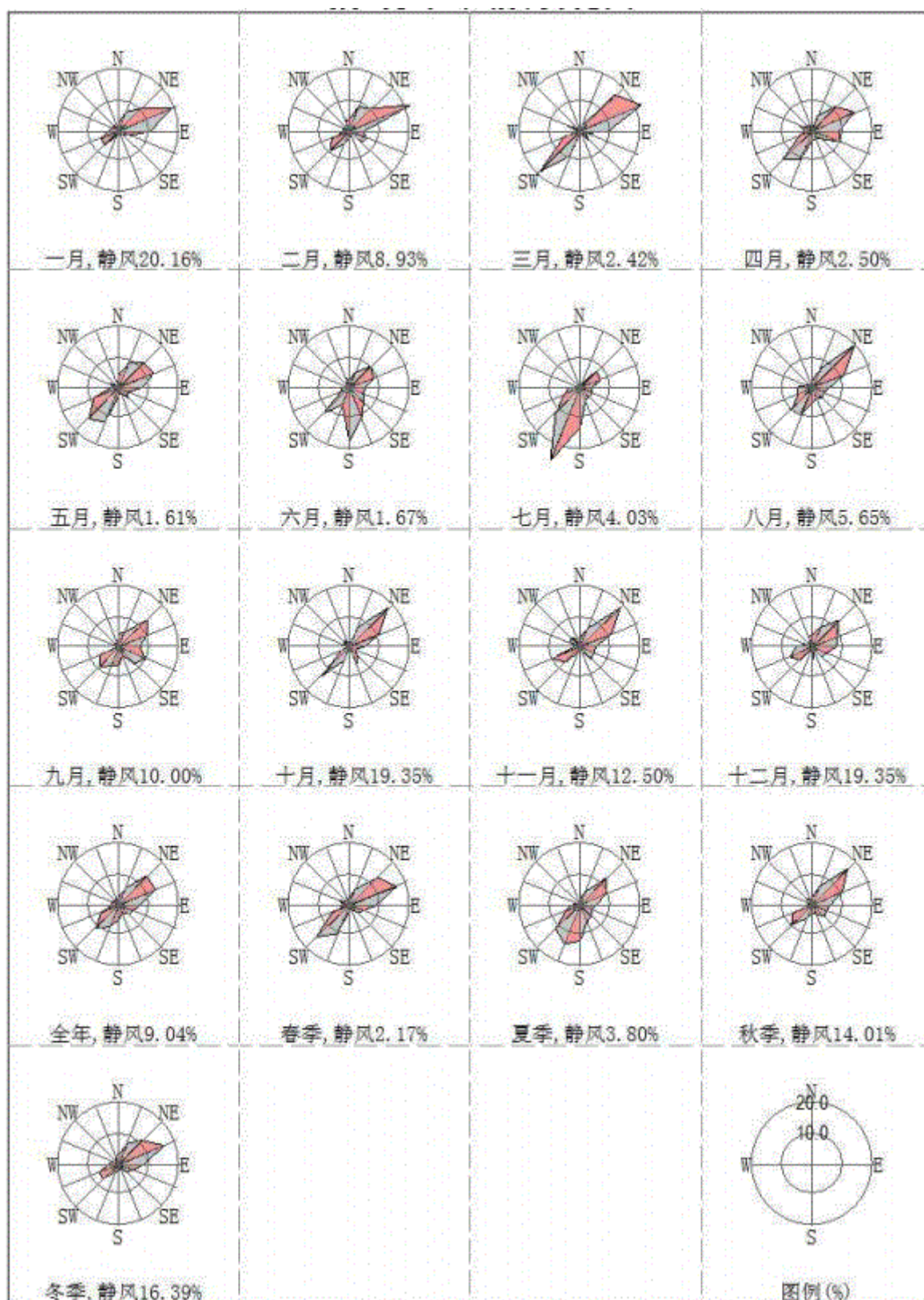
图5-4 唐河县2019年全年及各季风频玫瑰图
