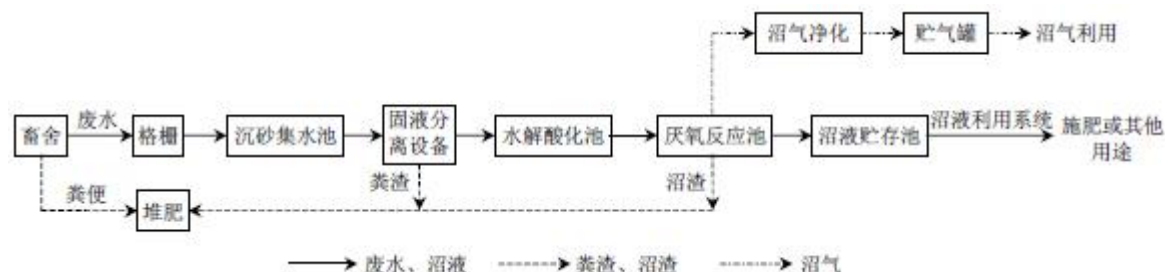
图6-1 模式II工艺基本流程
