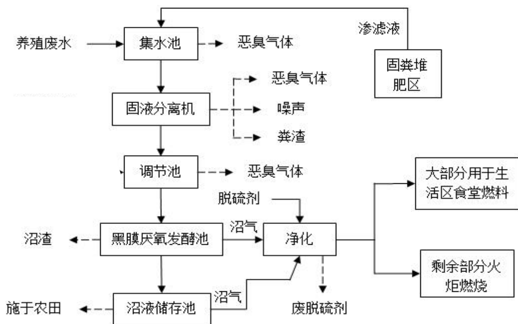
图 3-4 项目粪污处理工艺流程及产污环节示意图
