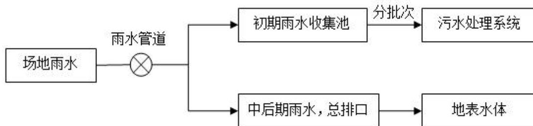
图 3-7 本工程初期雨水收集和排放示意图
