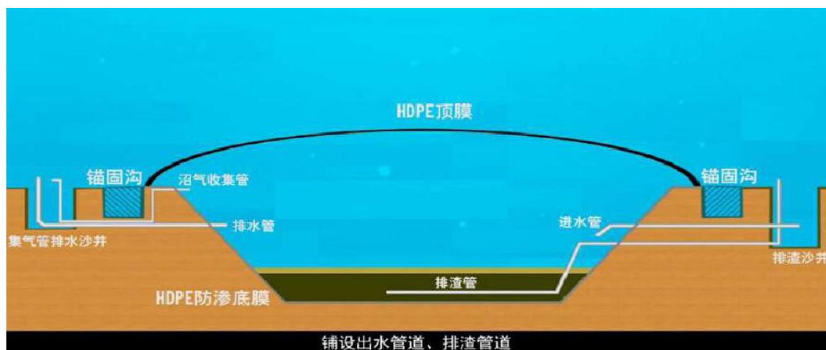
图6-3 全封闭黑膜厌氧发酵池结构示意图
