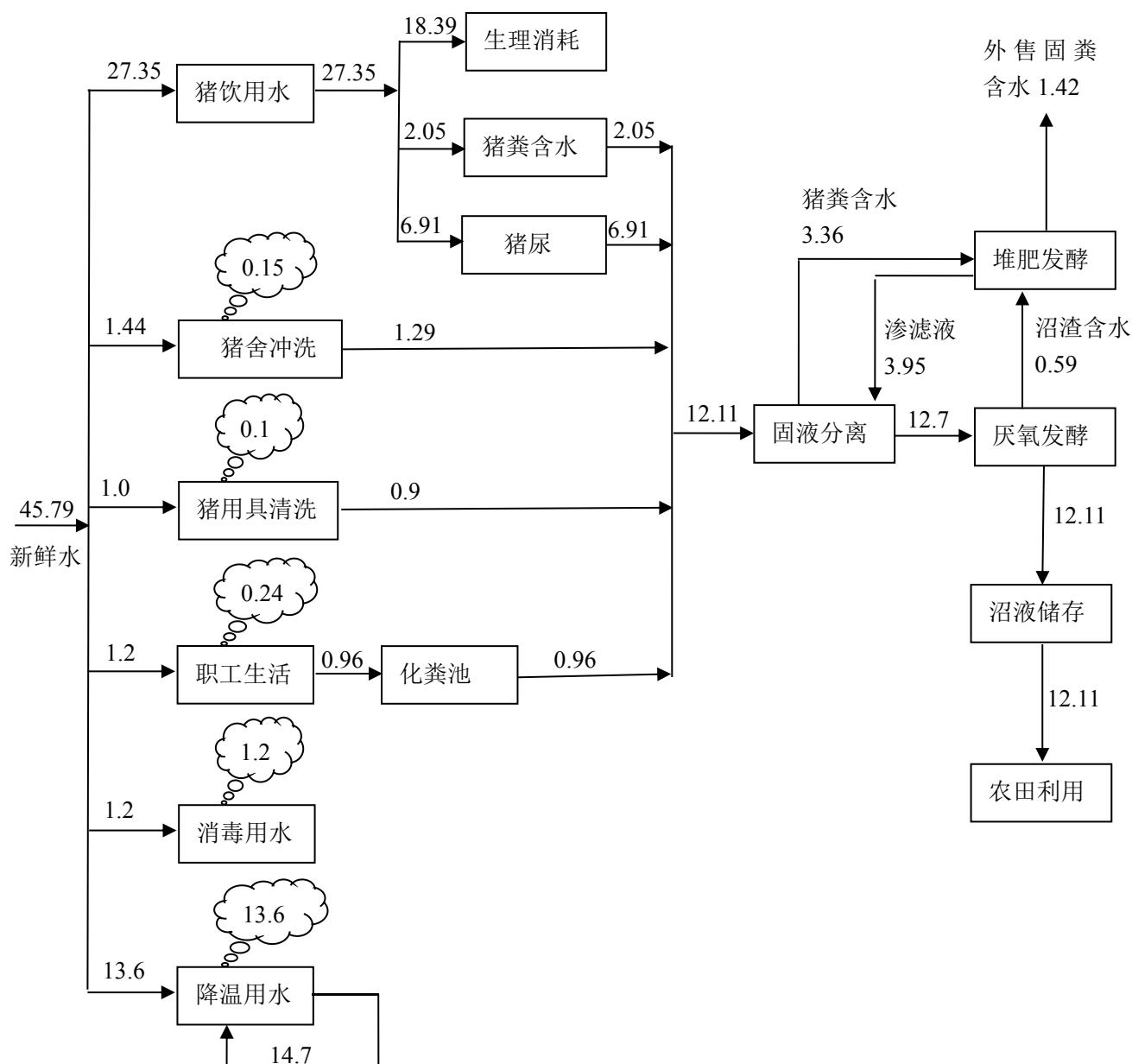
图 3-8 本项目水平衡图 (单位: \text{m}^3/\text{d} )
