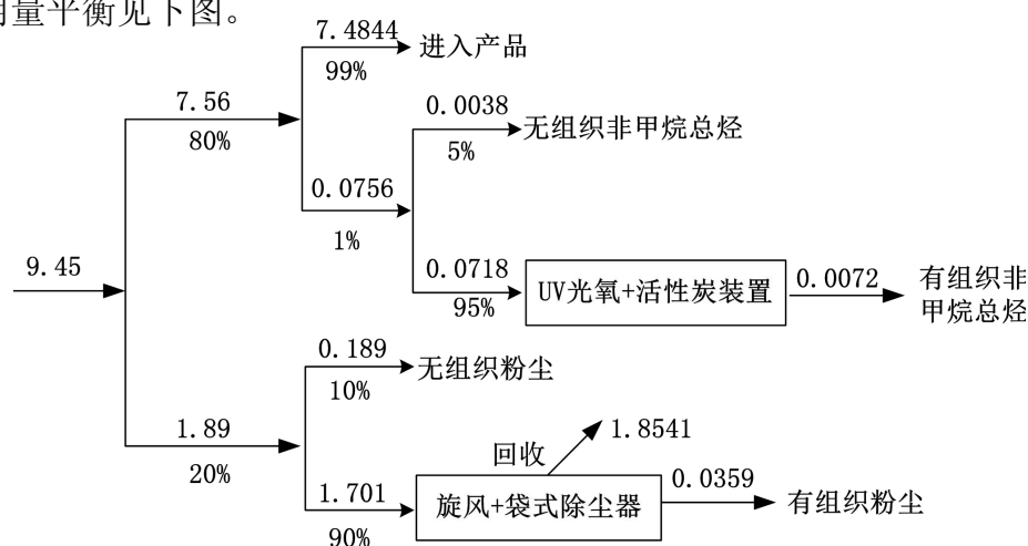
图 5 塑粉物料平衡图 (单位: t/a)
