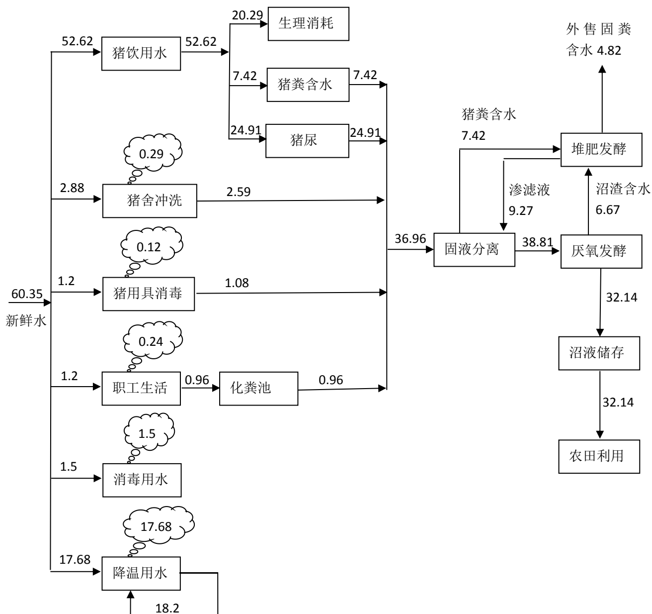
图 3-8 本项目水平衡图（单位：m³/d）
