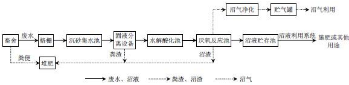
图6-1 模式II工艺基本流程
