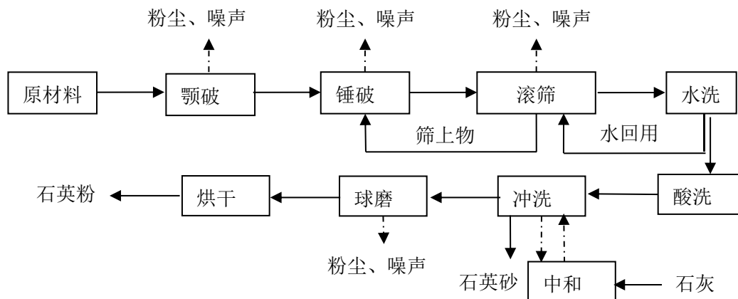
图 4 营运期生产工艺流程及产污环节
