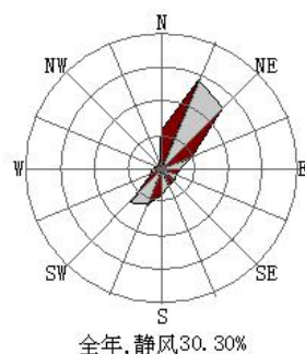
图 3 唐河县全年风频玫瑰图
