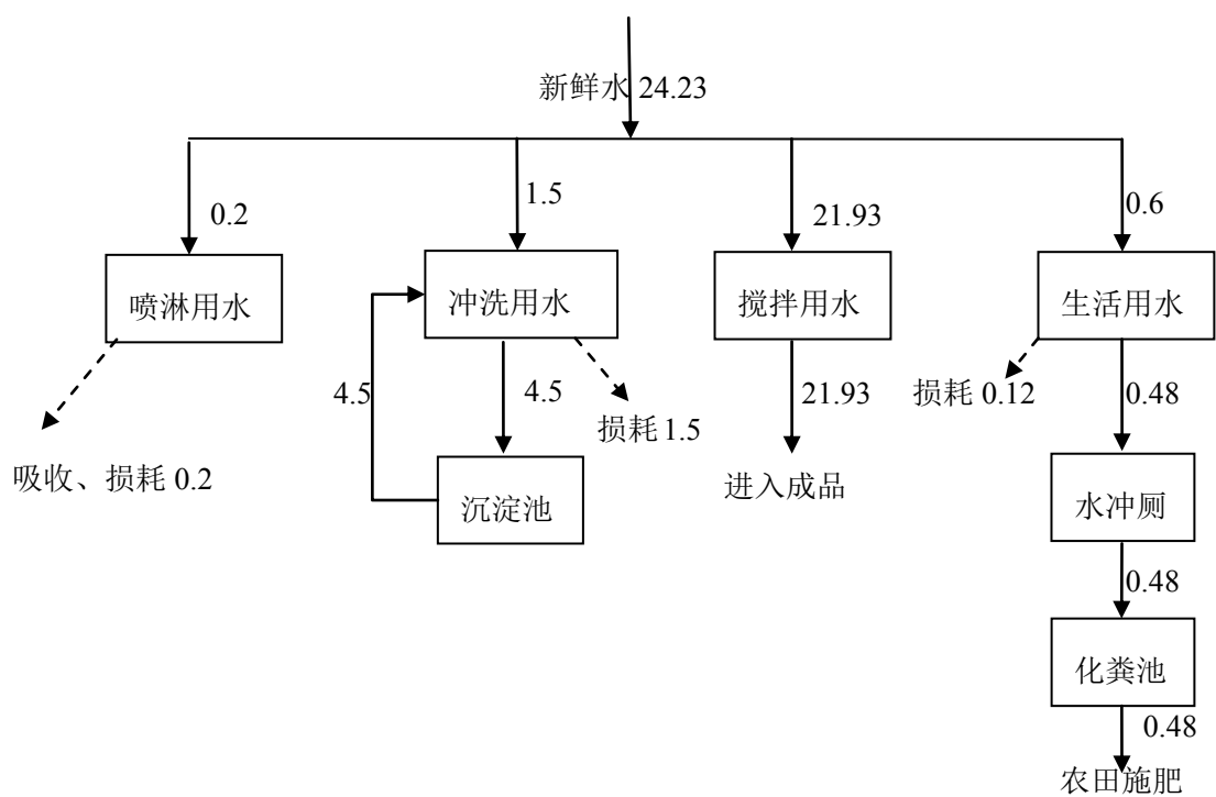
图 4 项目水平衡图 (m³/d)
