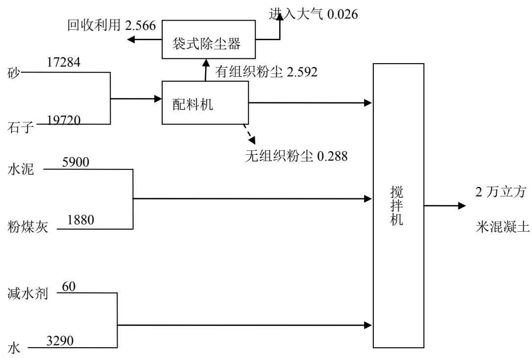
图 5 项目物料平衡图（单位 t/a）
