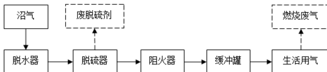
图3-4 沼气利用流程及产污环节示意图
