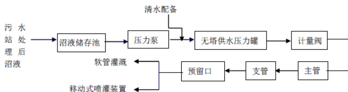
图6-6 沼液农田利用流程图
