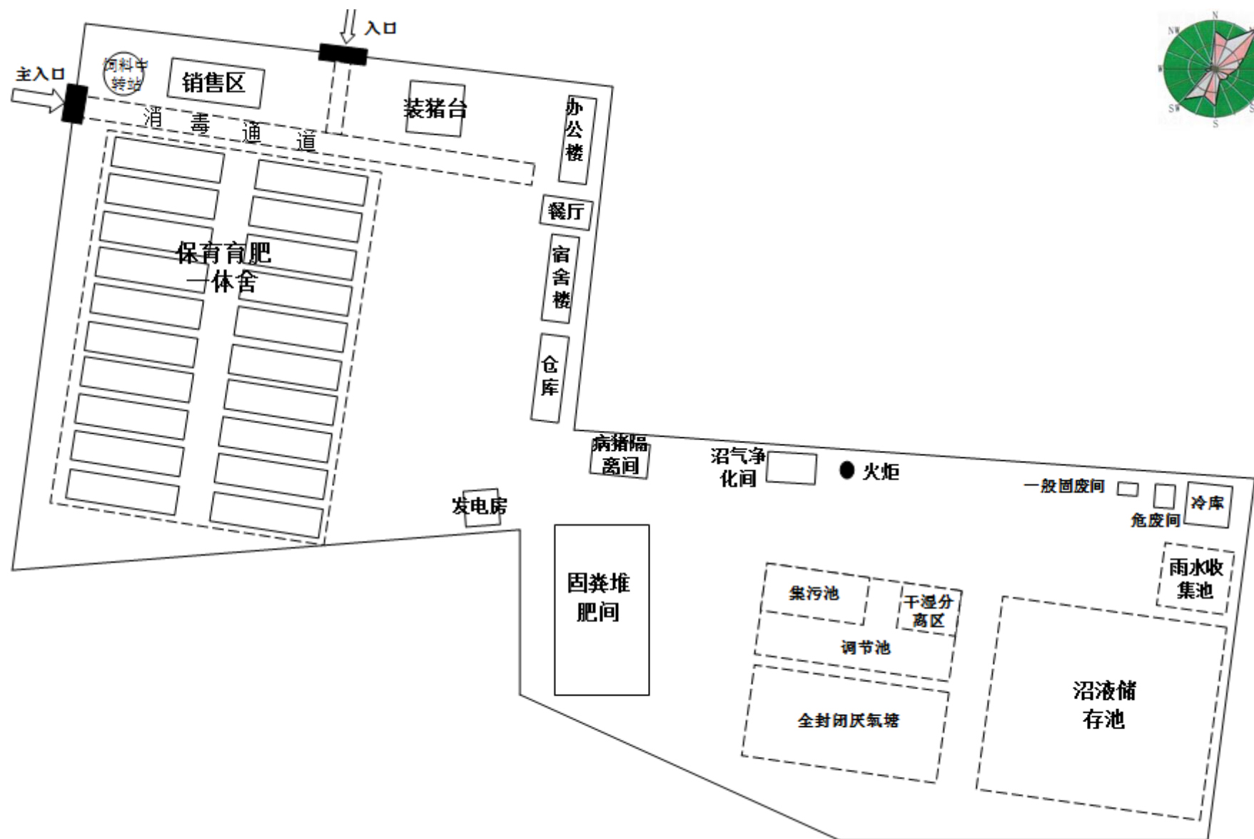
附图四 项目场区平面分布图
