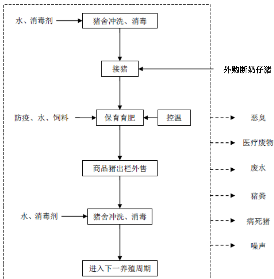
图3-1 保育育肥饲养流程及产污环节图
