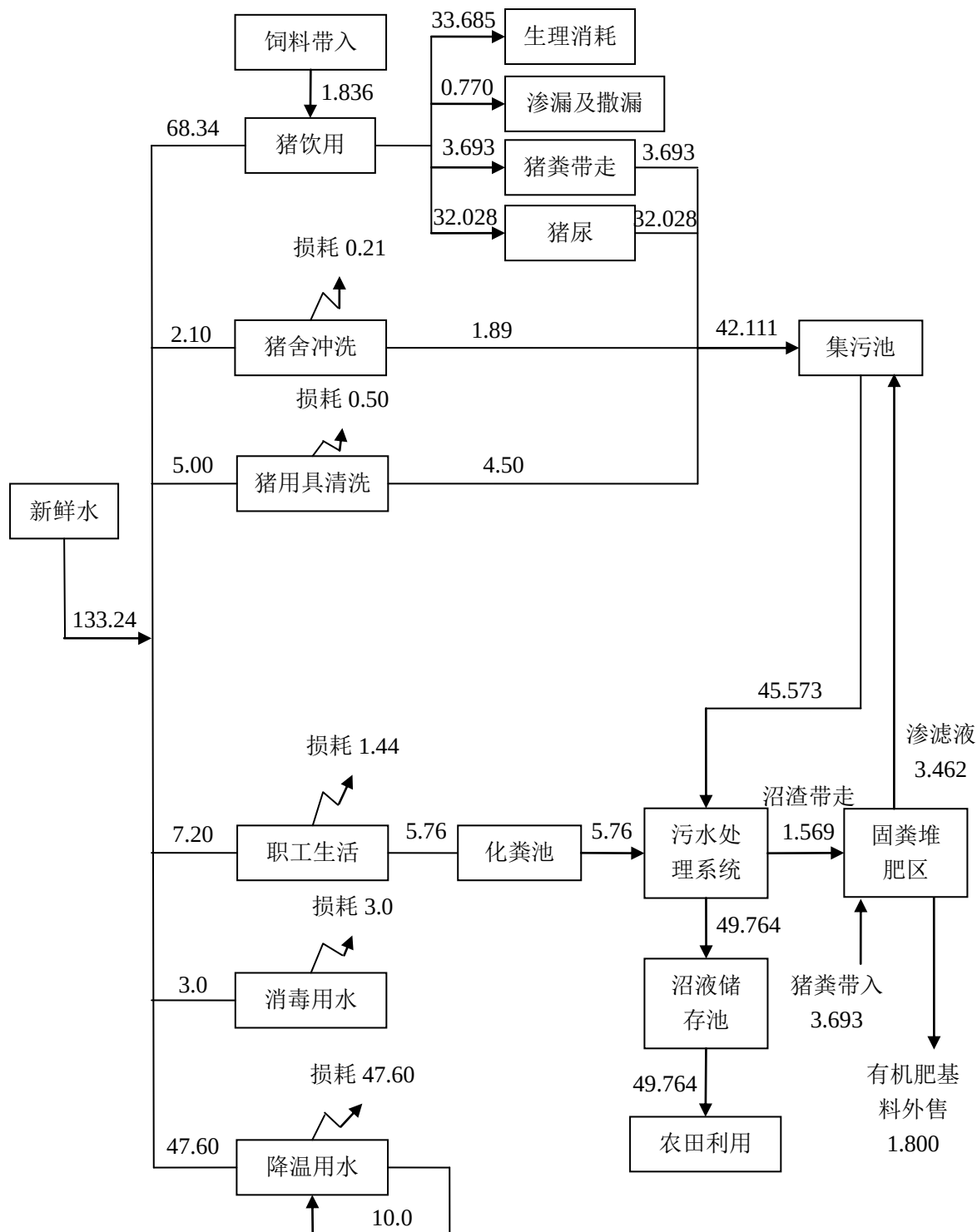
图3-7 本项目工程水平衡图 单位: \text{m}^3/\text{d}
