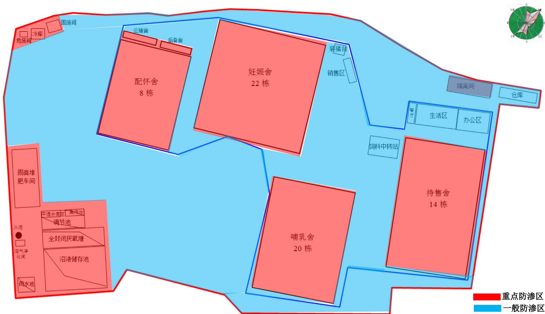
附图七 项目场区地下水分区防渗分布图
