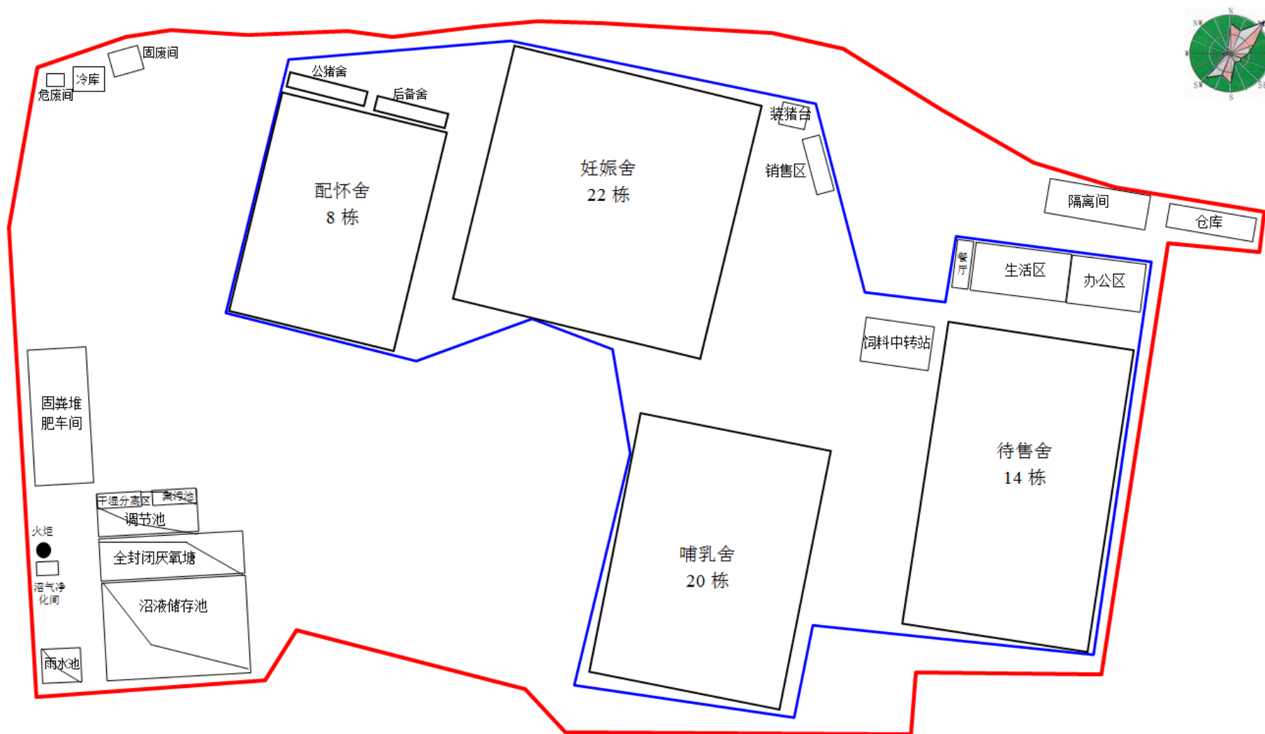
附图四 项目场区平面布置图
