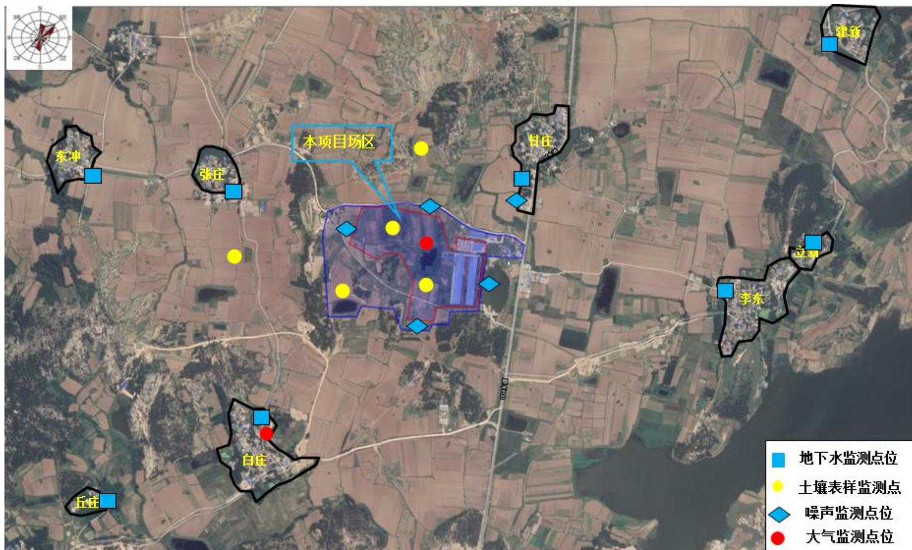
附图六 环境质量现状监测点位分布图（大气、地下水、土壤和噪声）
