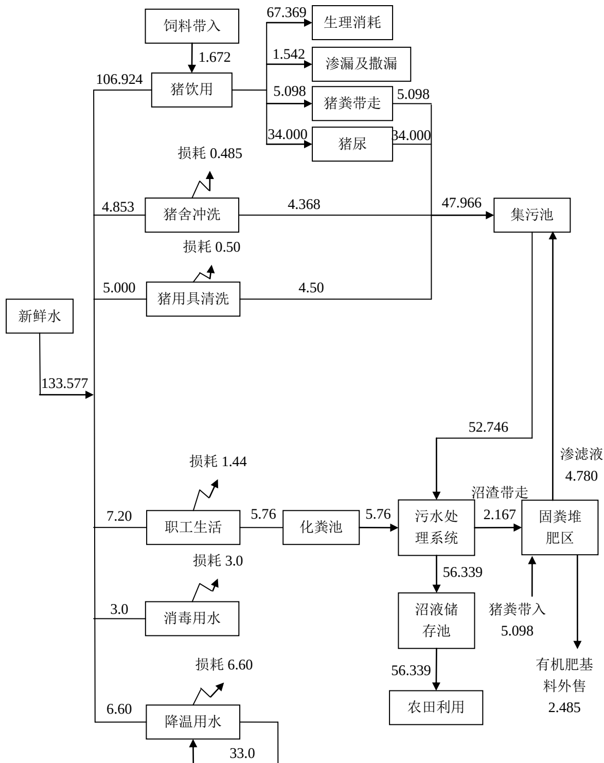
图3-7 本项目工程水平衡图 单位：m³/d
