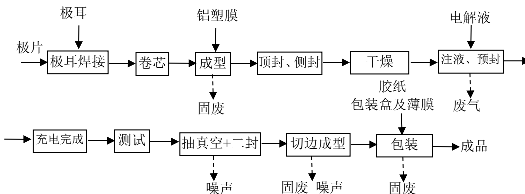
图 3 电池生产工艺流程及产污环节
