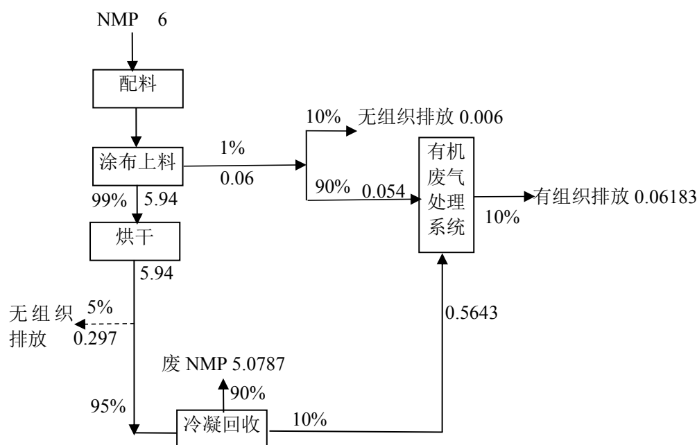
图 4 N-甲基吡咯烷酮物料平衡图 单位: t/a
