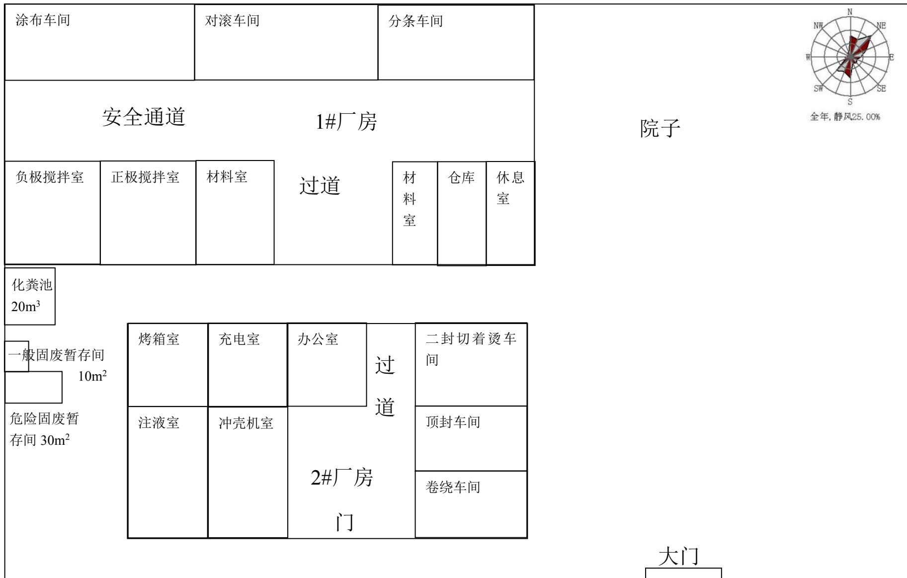
附图四 项目平面布置图
