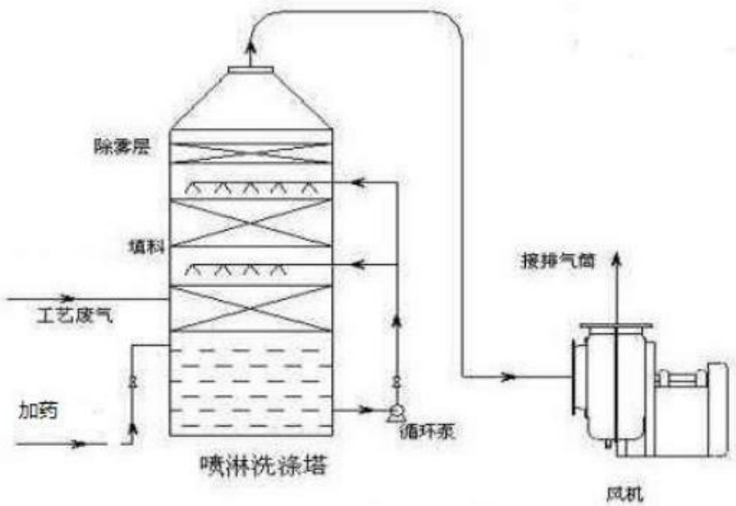
图 3 碱液喷淋净化系统工艺流程
