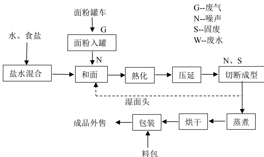
图5 冲泡面工艺流程图
