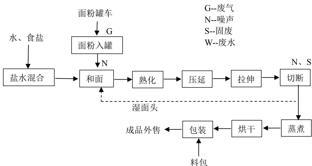
图4 自加热面工艺流程图
