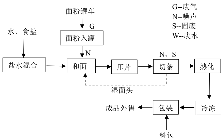
图5 冲泡面工艺流程图
