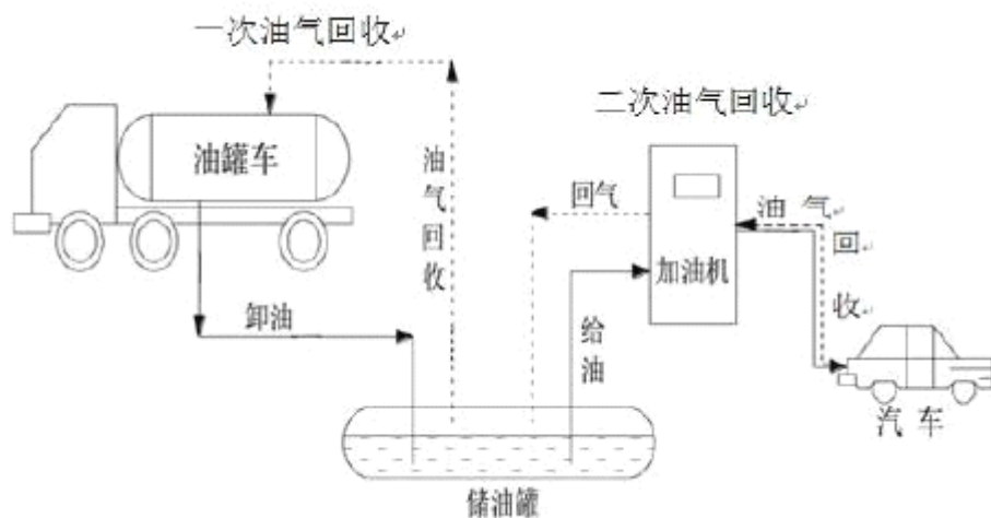
图 2-4 加油站工艺流程图
