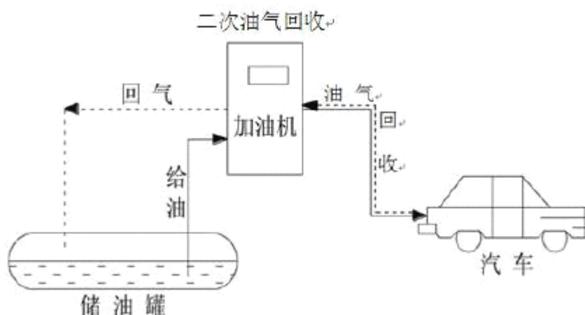
图 2-3 成品油加油工艺流程图
