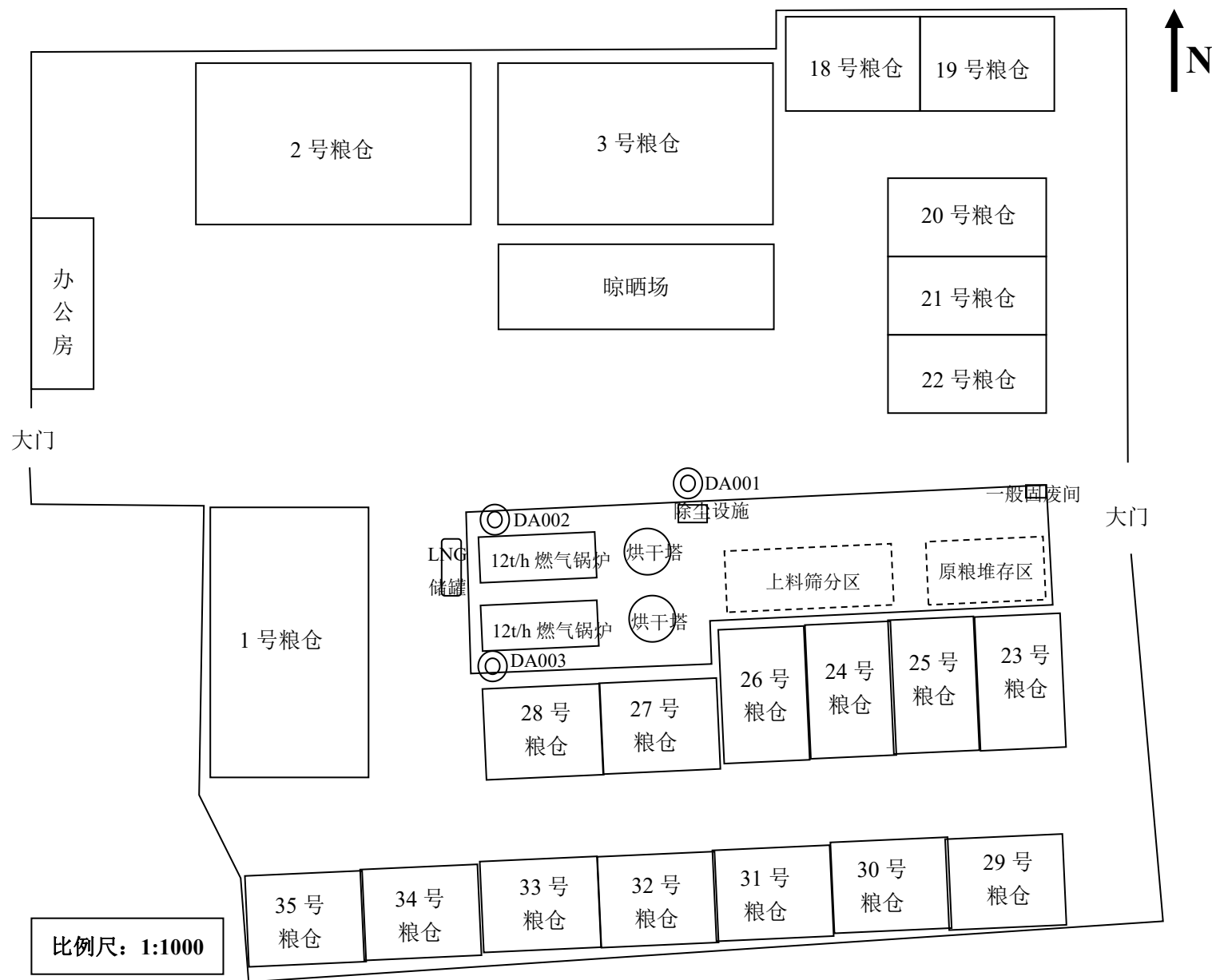
附图 2 项目厂区平面布置图
