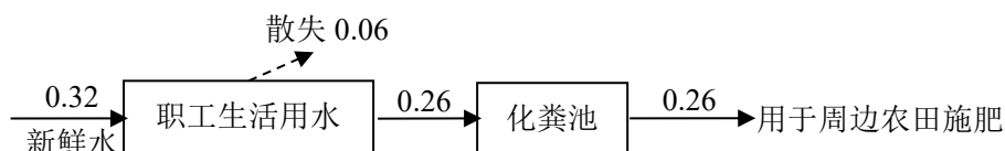
图 2-1 项目营运期水平衡图 单位：m 3 /d
