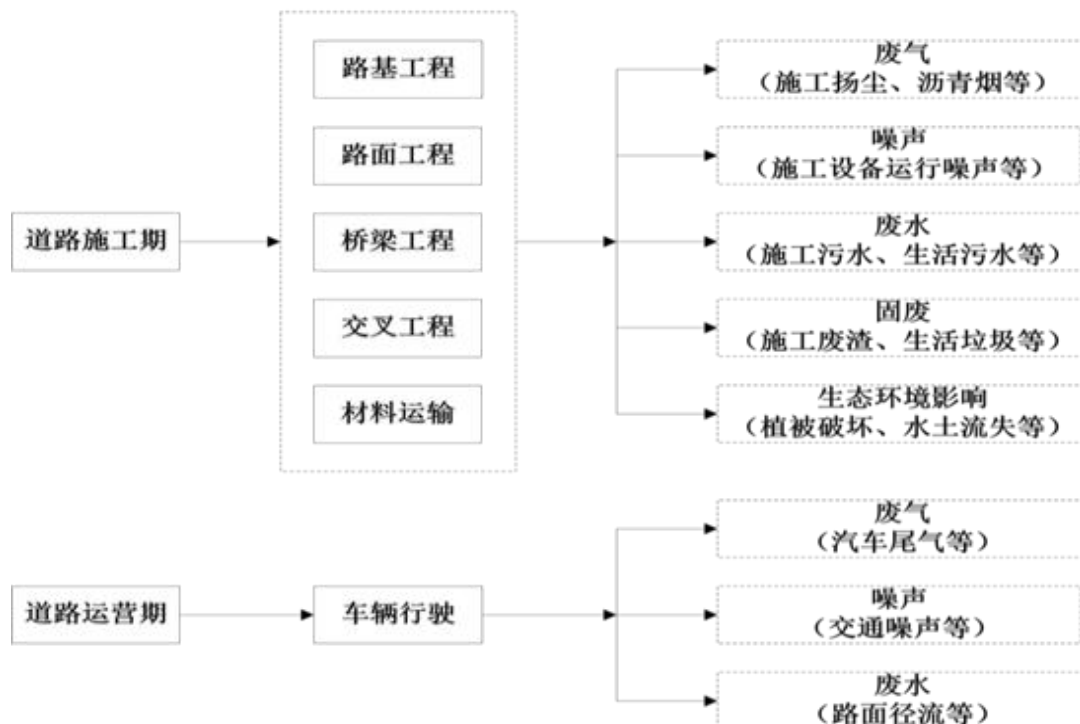
图3 项目施工及运营期工艺流程及产污分析图
