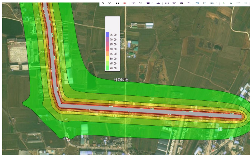
(1) 起点路段近期昼间水平方向等声级线 (马振抚镇)
