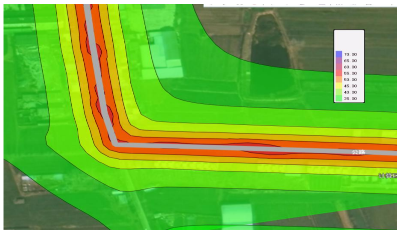
(1) 起点路段中期昼间水平方向等声级线 (马振抚镇)
