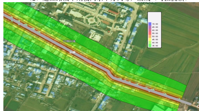
(4) 终点路段中期夜间水平方向等声级线 (咎岗镇)
