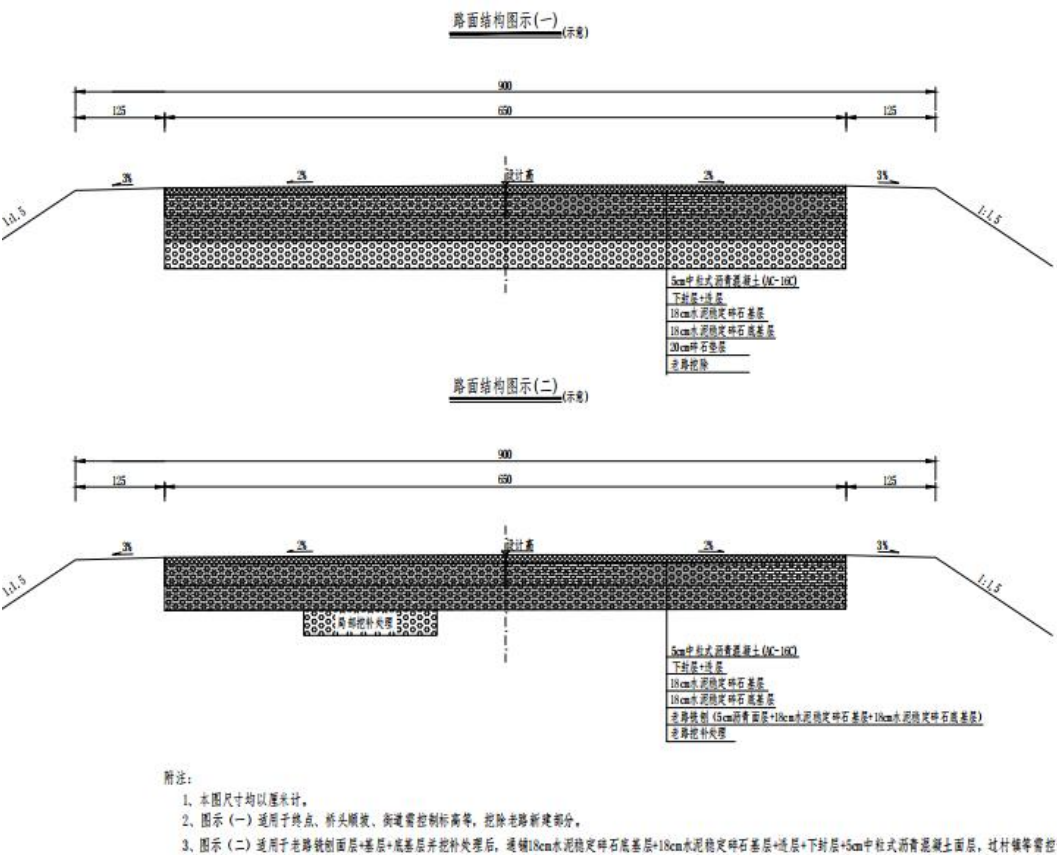
图 2 本项目路面结构图
