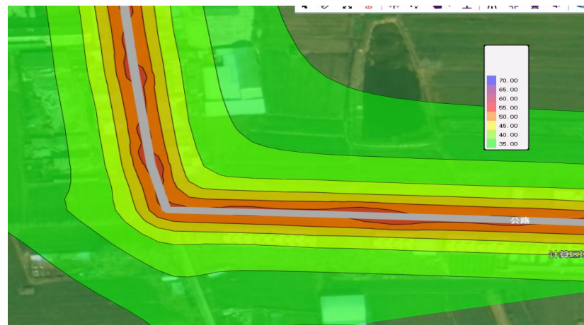
(2) 起点路段中期夜间水平方向等声级线 (马振抚镇)
