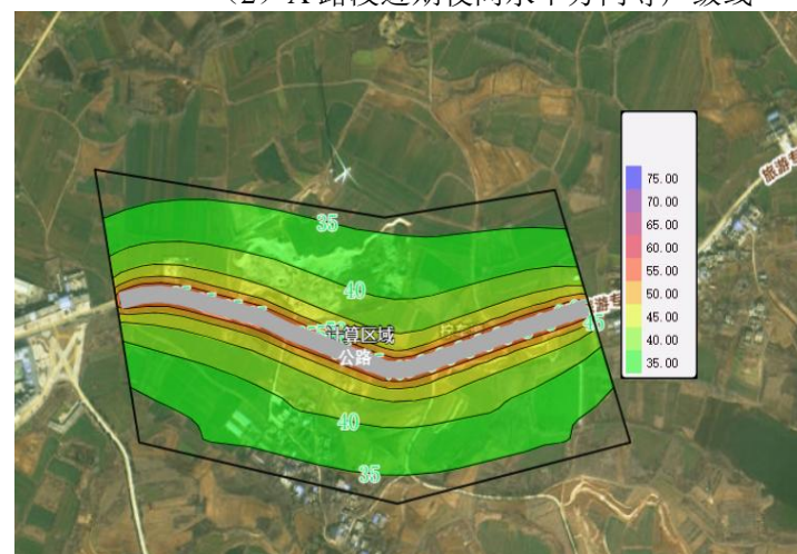
(4) A 路段中期夜间水平方向等声级线
