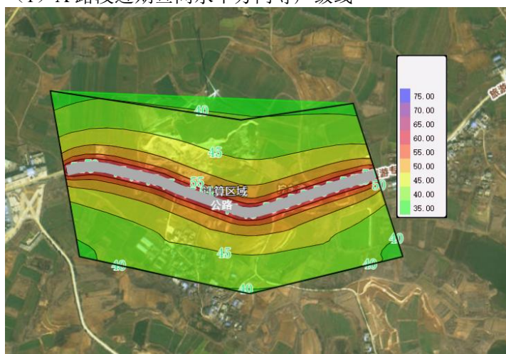
(3) A 路段中期昼间水平方向等声级线
