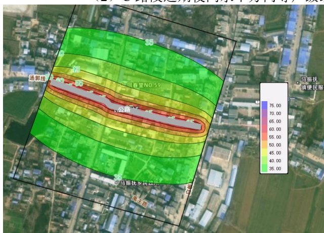
(4) C 路段中期夜间水平方向等声级线
