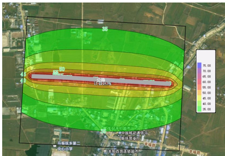
(1) B 路段近期昼间水平方向等声级线
