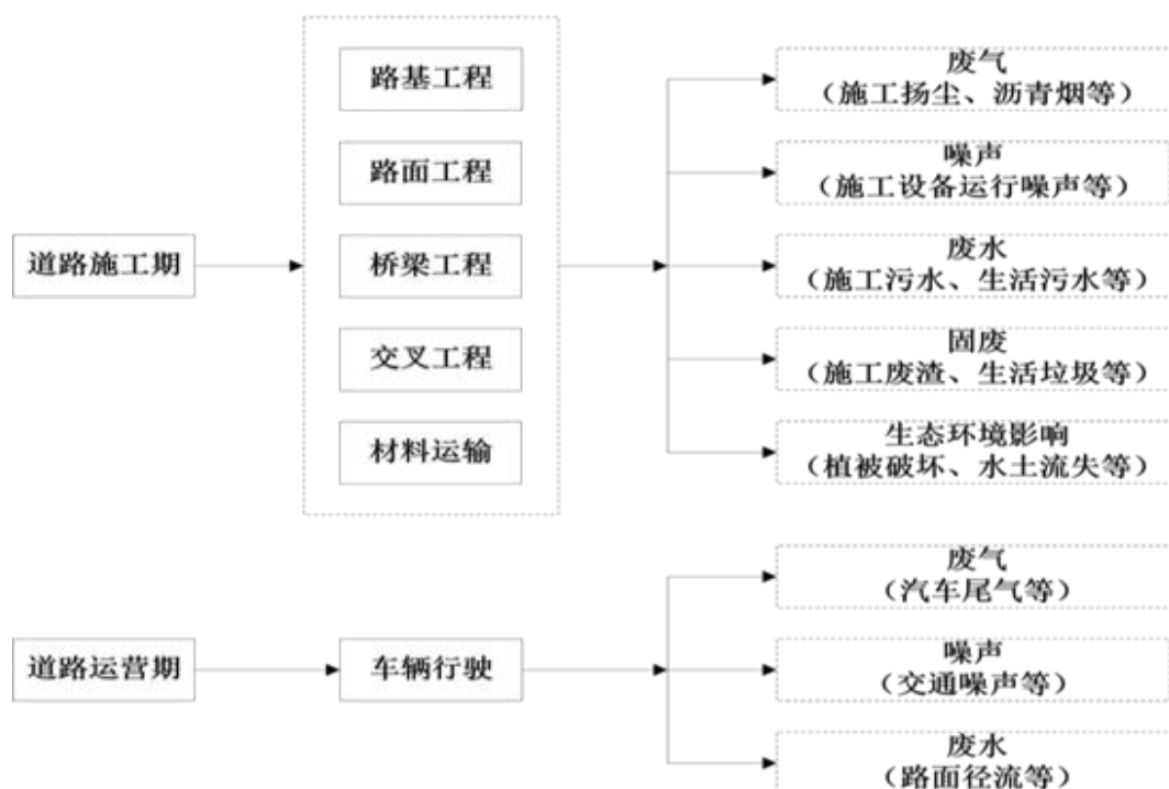
图4 项目施工及运营期工艺流程及产污分析图
