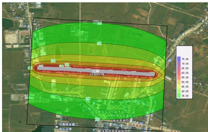
(3) B 路段中期昼间水平方向等声级线
