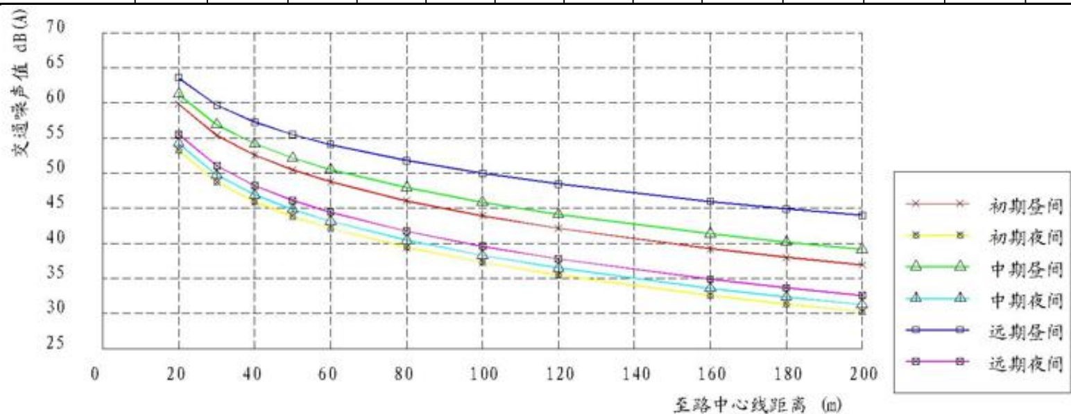
图 1.7 本项目营运期交通噪声污染曲线图
