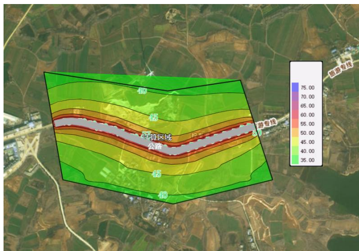
(1) A 路段近期昼间水平方向等声级线
