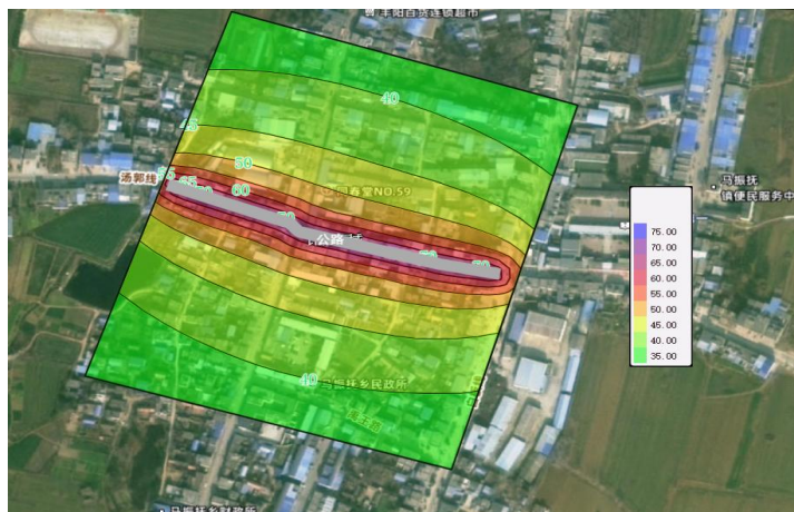
(1) C 路段近期昼间水平方向等声级线
