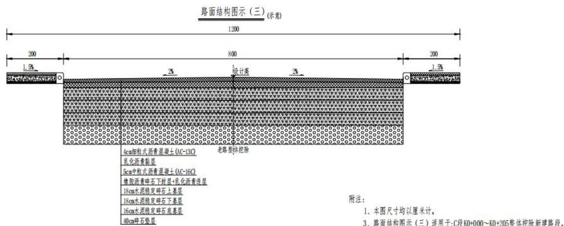
图 3 本项目路面结构示意图
