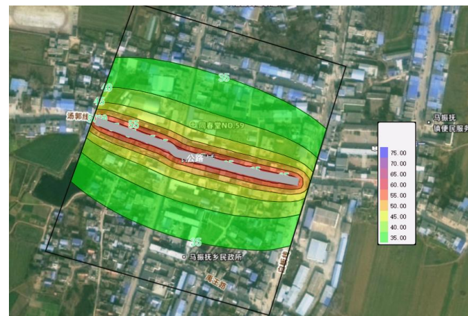
(2) C 路段近期夜间水平方向等声级线
