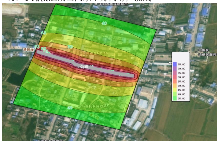
(3) C 路段中期昼间水平方向等声级线
