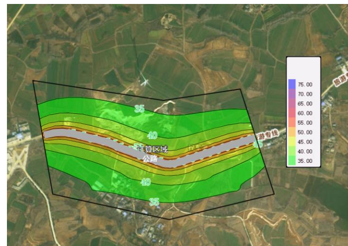
(2) A 路段近期夜间水平方向等声级线
