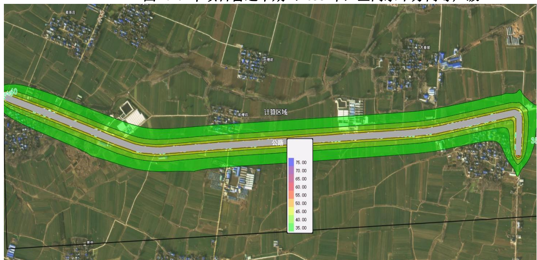
图 1.11 本项目营运中期（2033 年）夜间水平方向等声级
