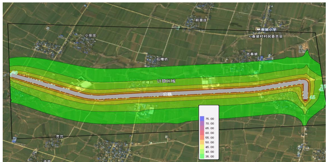
图 1.12 本项目营运远期（2041 年）昼间水平方向等声级
