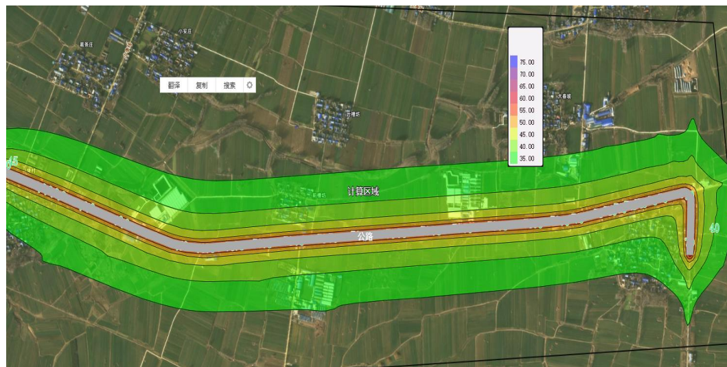
图 1.8 本项目营运近期（2027 年）昼间水平方向等声级
