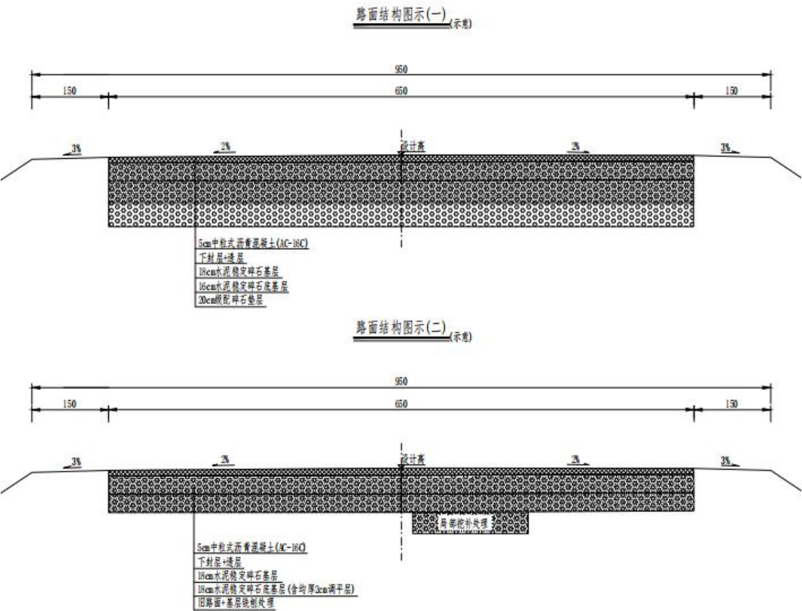
图 2 本项目路面结构示意图
