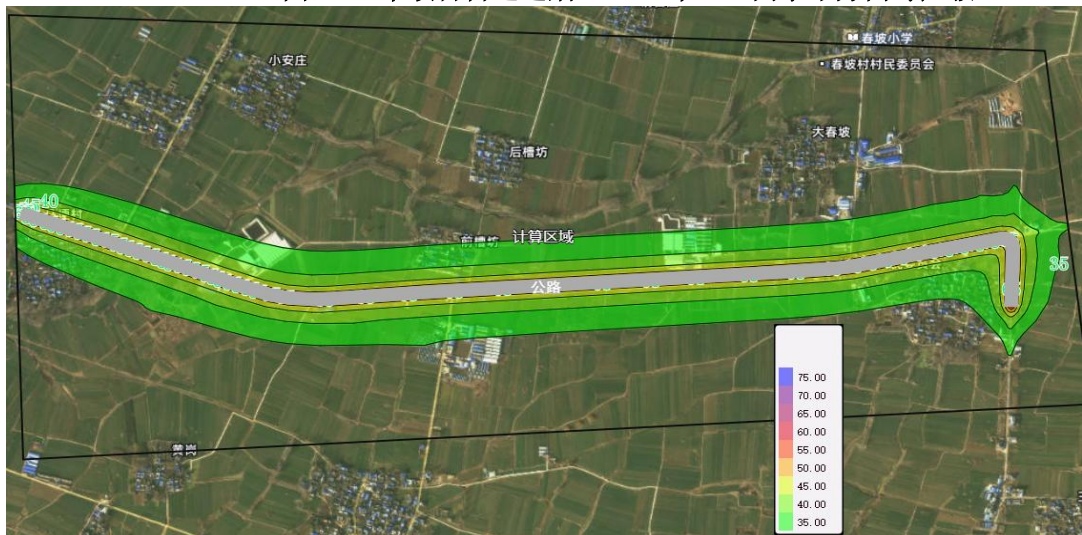
图 1.13 本项目营运远期（2041 年）夜间水平方向等声级
