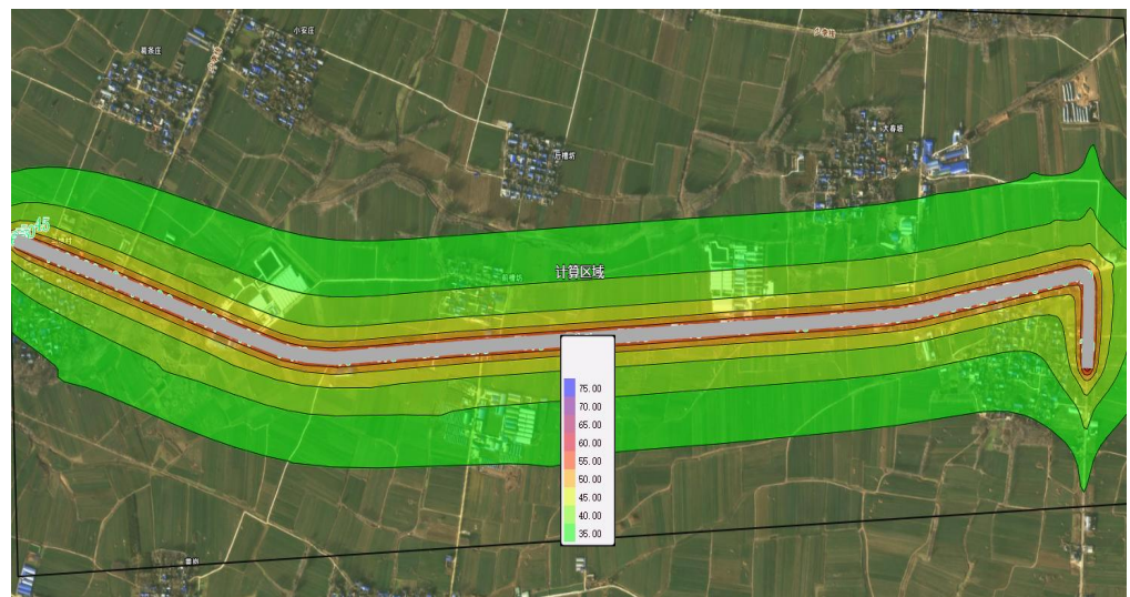
图 1.10 本项目营运中期（2033 年）昼间水平方向等声级
